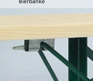
Arretierung Biertisch und Bierbänke
